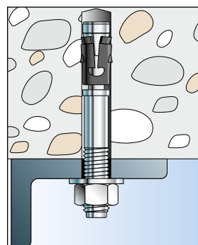
Goujon d'ancrage FAZ II Plus
