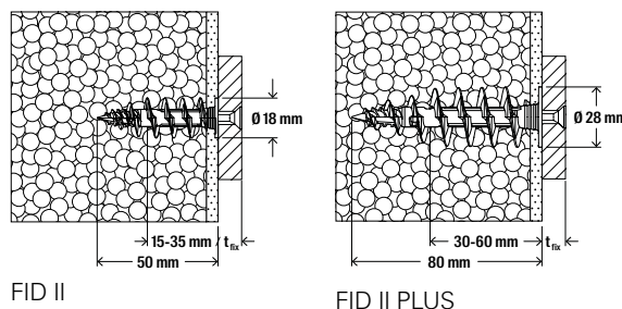
Fixation sur isolant FID II Plus
