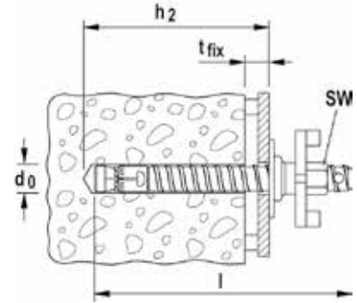
Ensemble de fixation pour carotteuse FDBB
