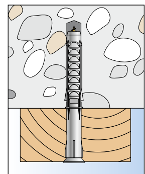
Cheville rallongée SXS
