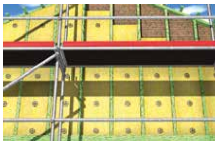
Isolants sur façades ventilées
