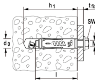
Cheville pour charges lourdes TA M-S avec vis
