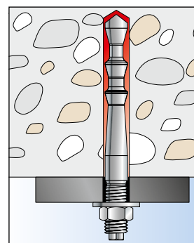
Ancre scellé avec cône
